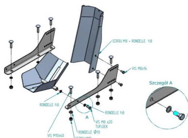
Bloque roue pour moto permet de tenir la moto droite pour la sangler sans avoir besoin de la mettre sur la béquille. Réf :K150.4141
